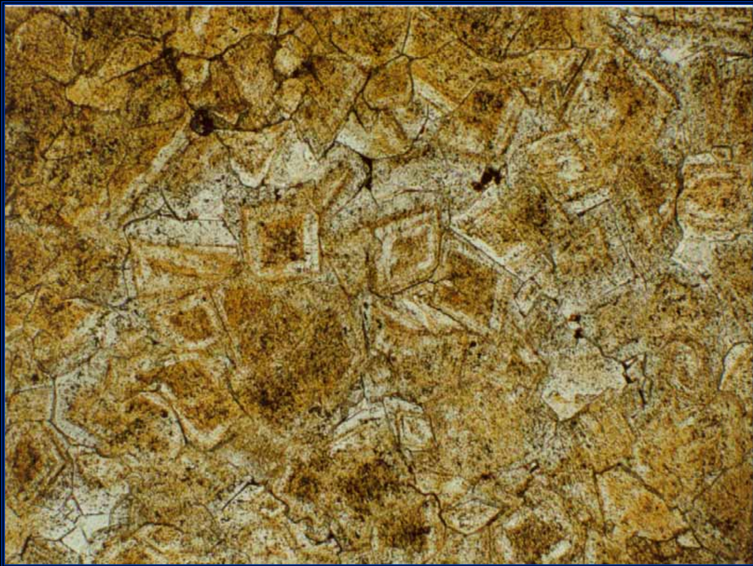
交代残余的“雾心亮边”菱面体白云石
